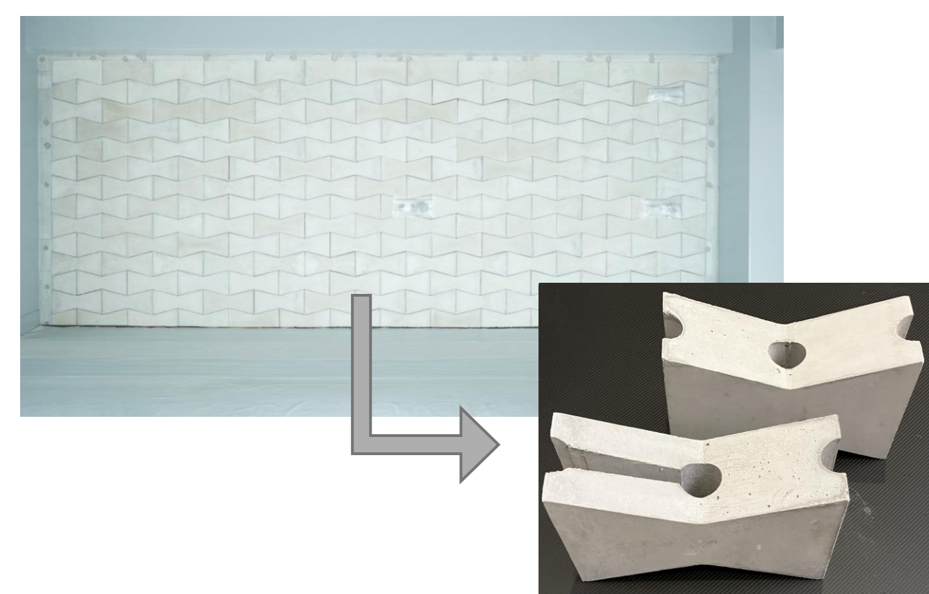
CUCO®-耐震補強用PCaブロック
