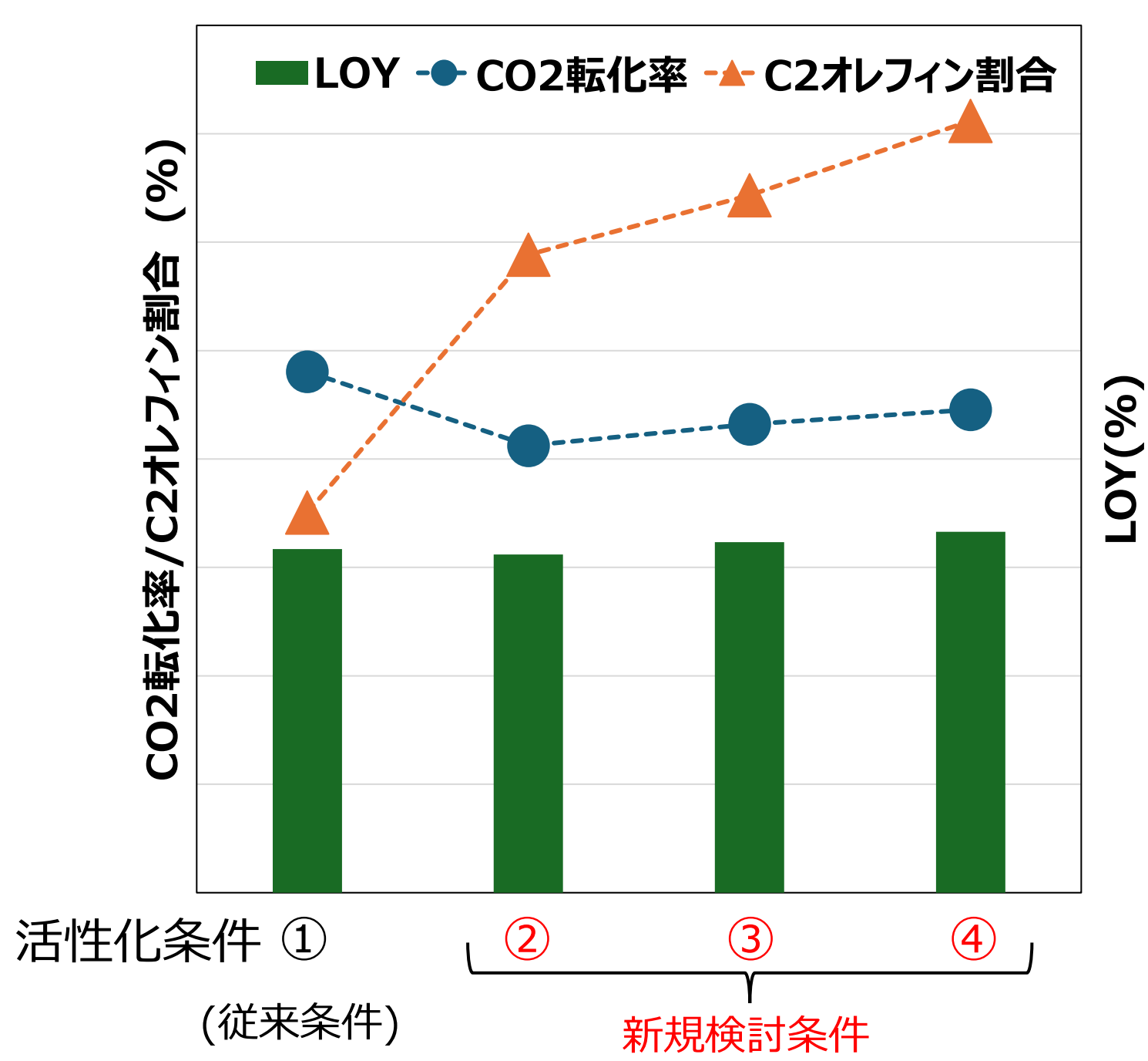
成形触媒を用いたラボ試験による性能試験
