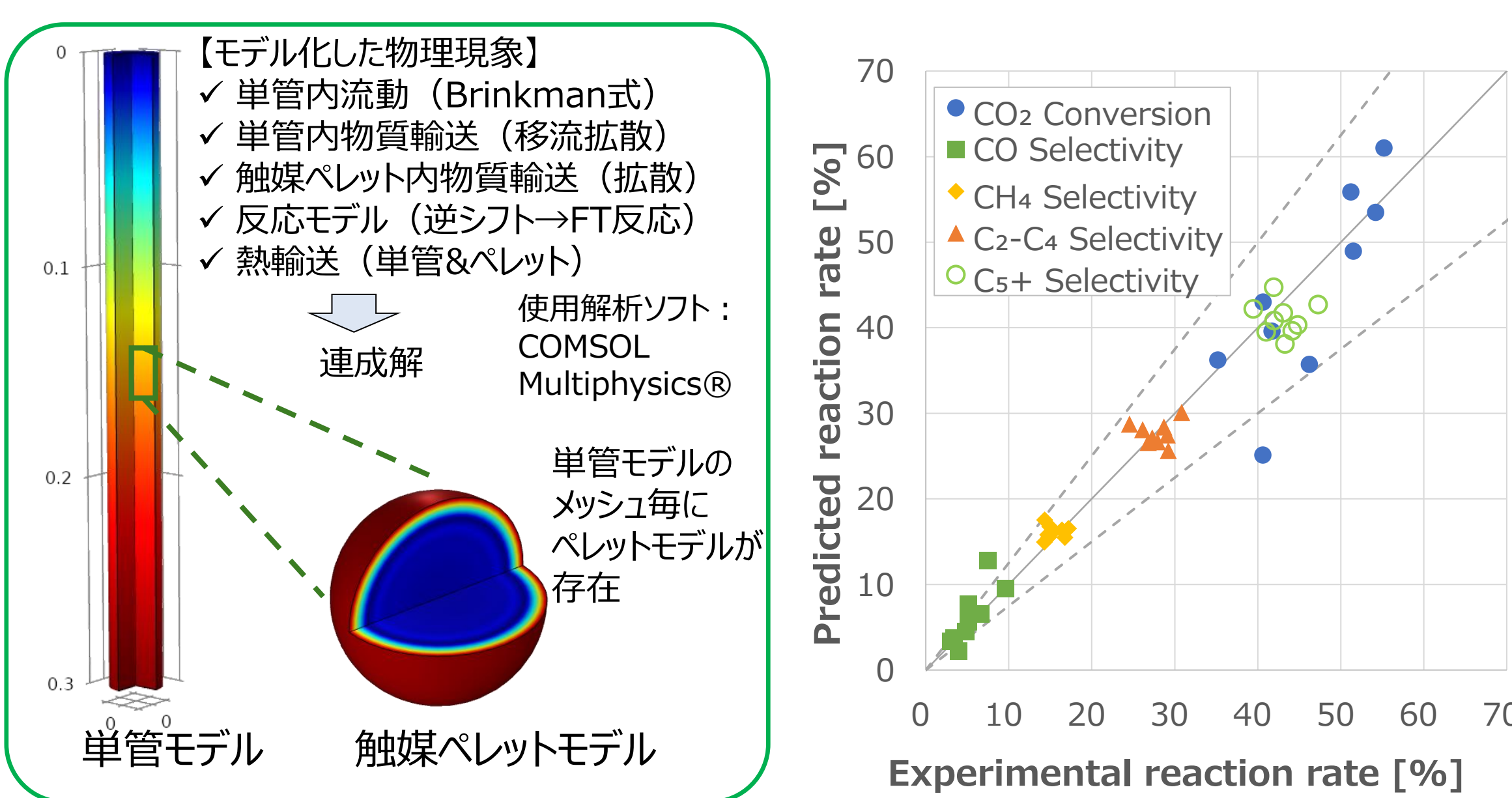
シミュレーションを活用した反応器開発
