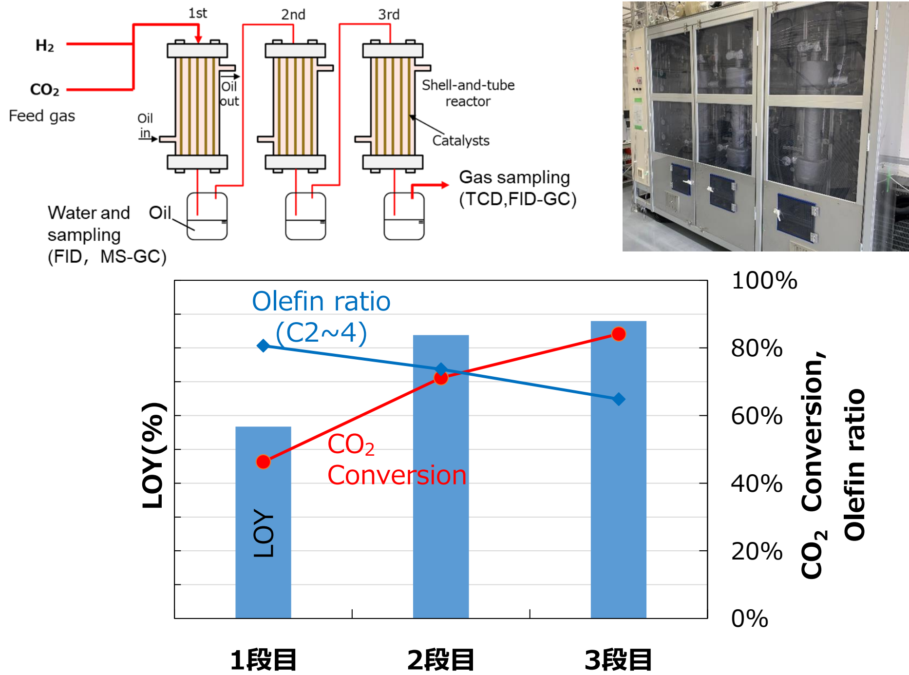
マルチステージリアクターによる性能向上検討
