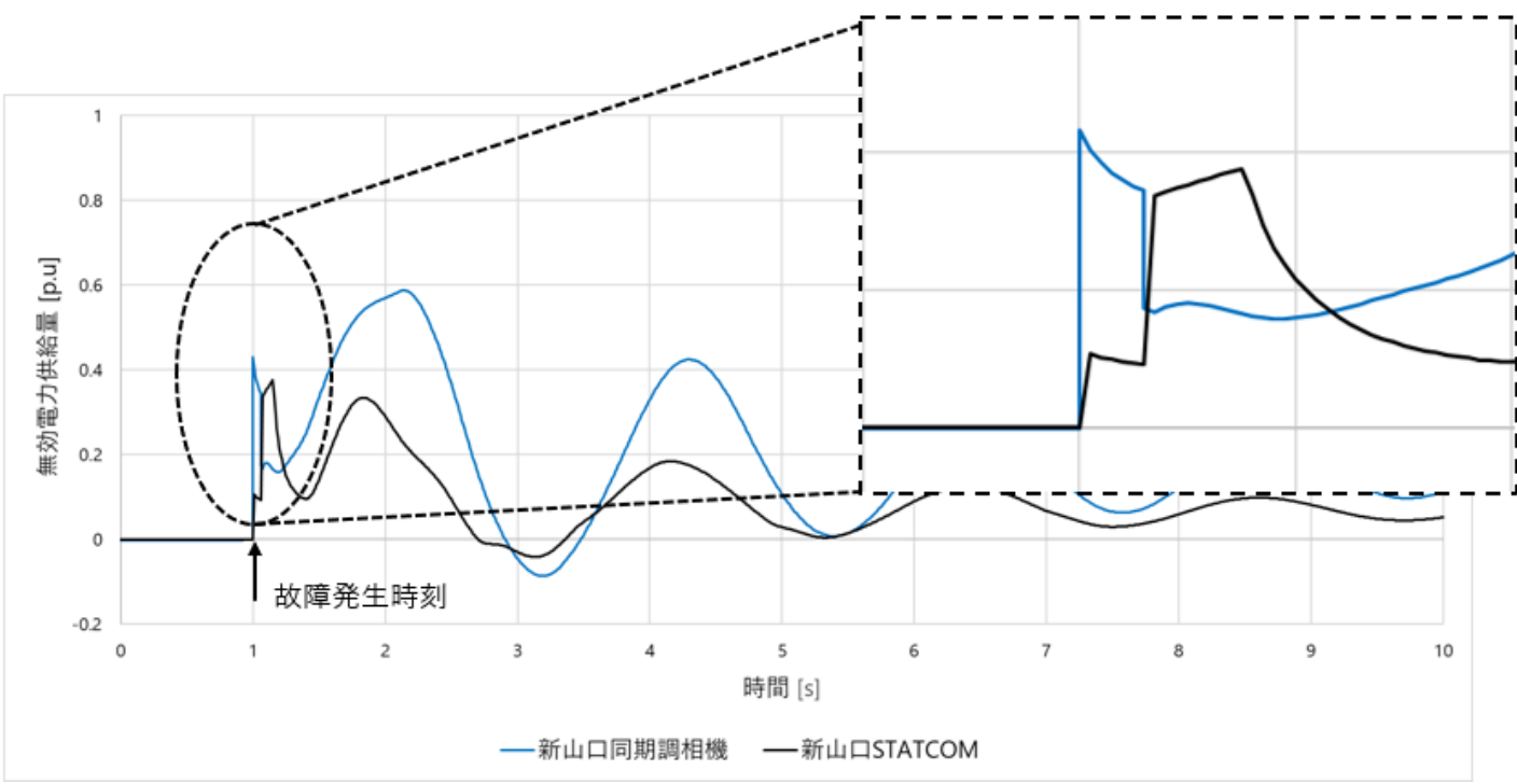
図6 無効電力供給量の比較
