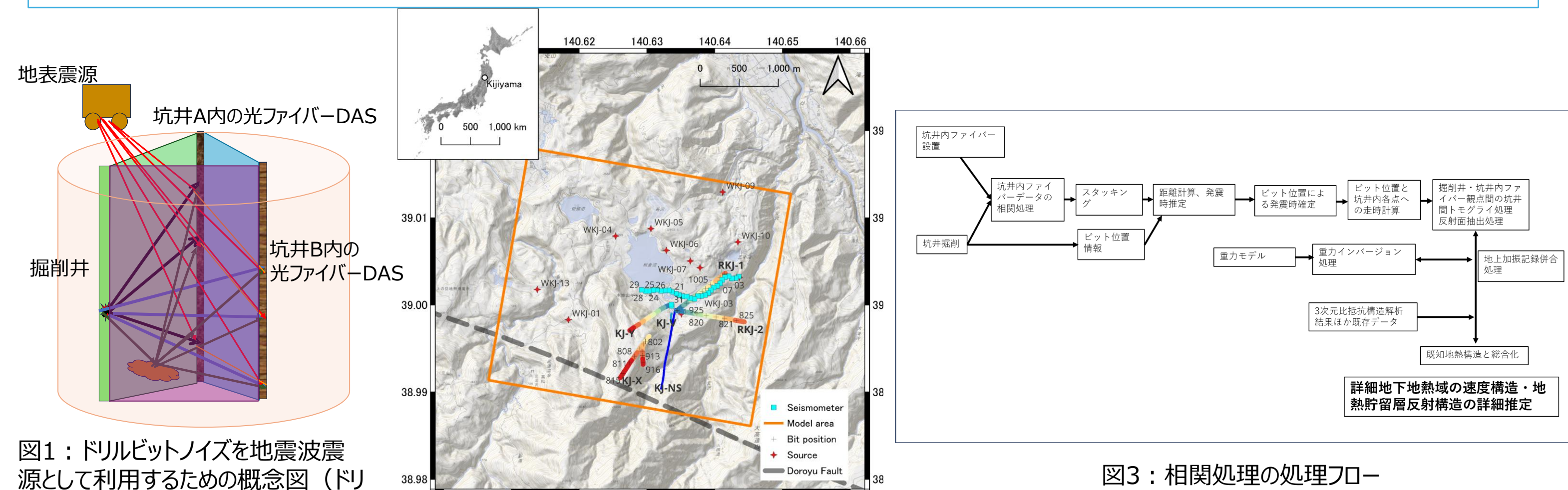
図2：本調査に用いた木地山での地熱坑井位置
