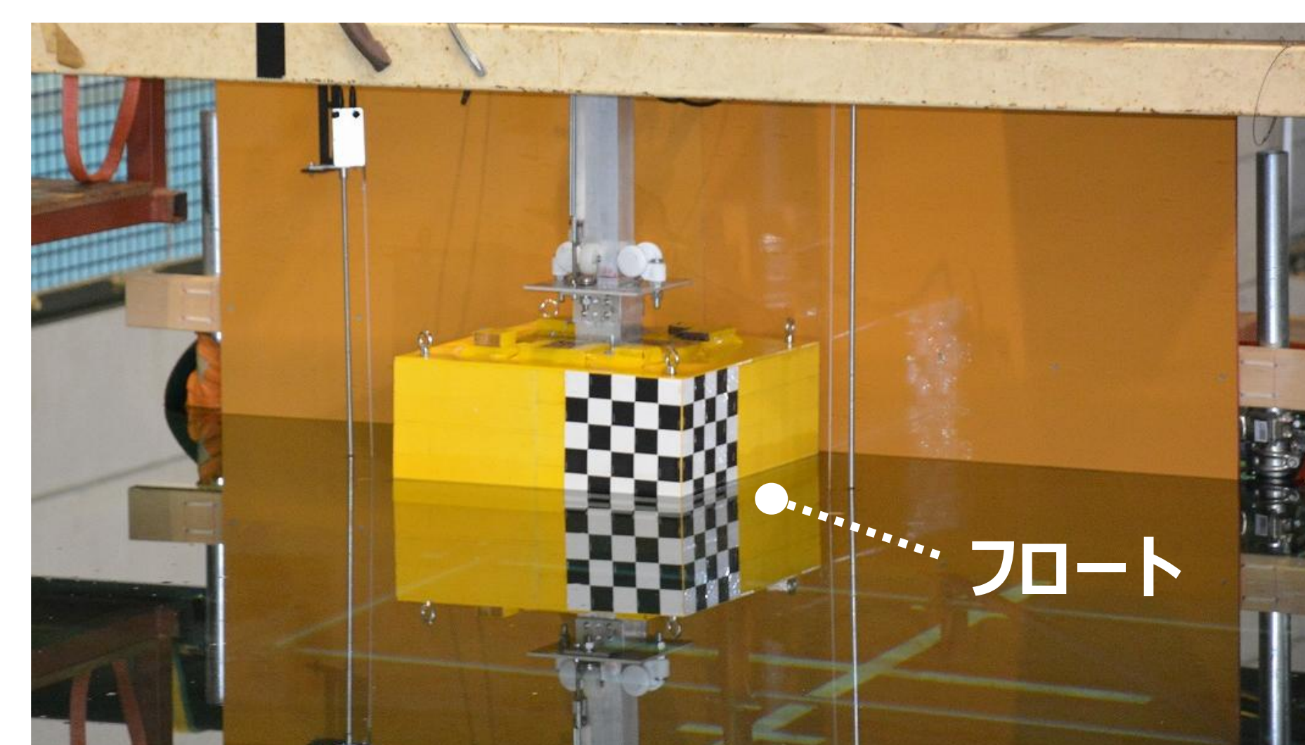
模型水槽試験
