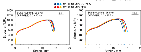
図 Stress-Stroke曲線
