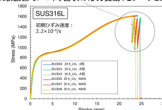
図 Stress-Stroke曲線
