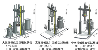
図 特殊実験施設外観および評価試験設備イメージ
