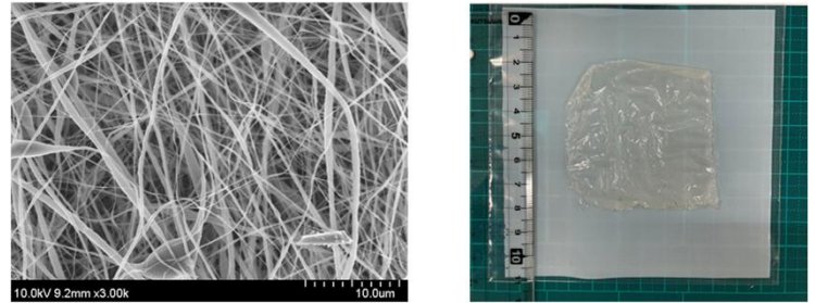
図2 PVDF-クエンチャー微多孔膜の電子顕微鏡観察結果（左図）とNafionハイブリッド電解質膜（右図）
