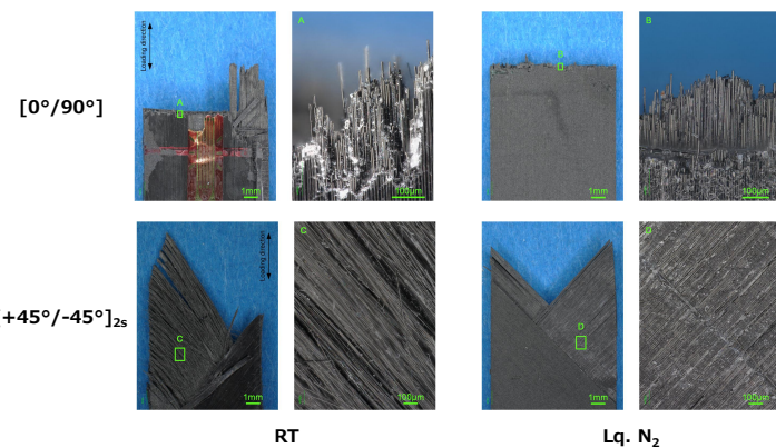
RT Lq. N2 破断部 引張試験 T700/#2592
