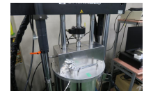
クライオスタット、液面計と 自動供給装置を導入
