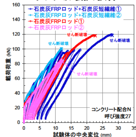
せん断破壊試験体
