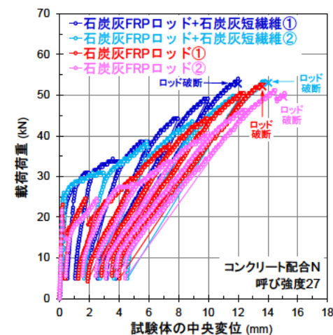
曲げ破壊試験体
