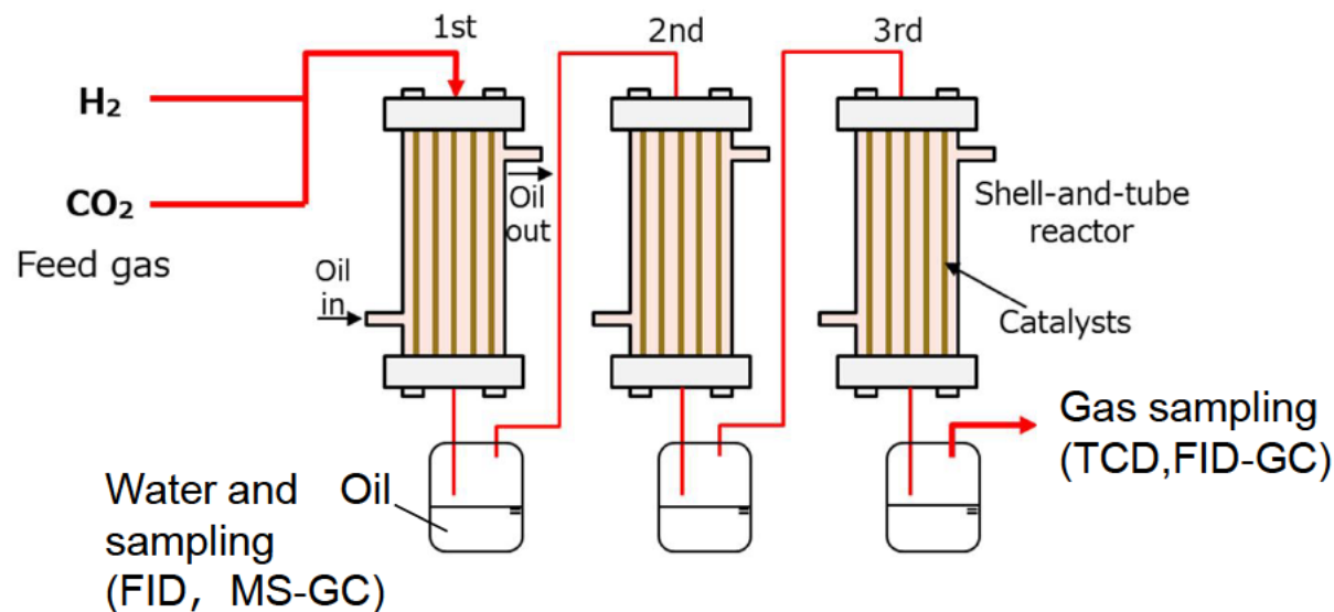
【多段式反応装置の概要図】
