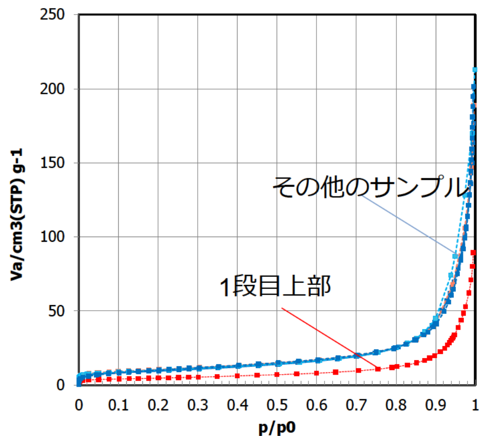
吸着等温線
