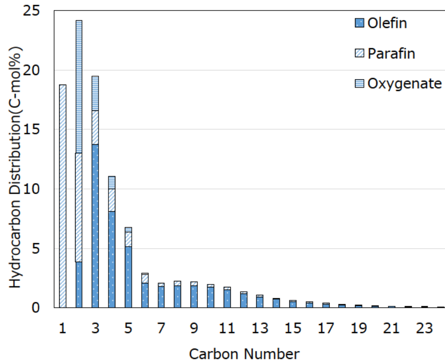
炭素数分布
