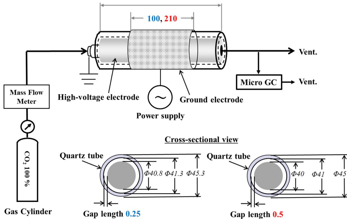
図1 CO 2 プラズマ分解実験装置
