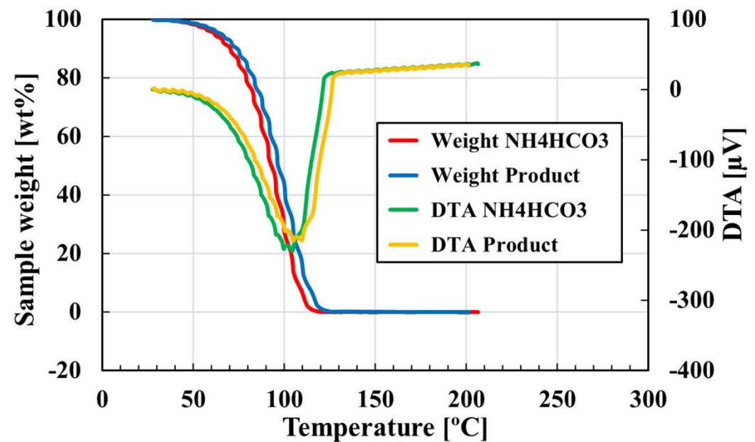
図 反応生成物と試薬(NH 4 HCO 3 )のTG-DTA結果
