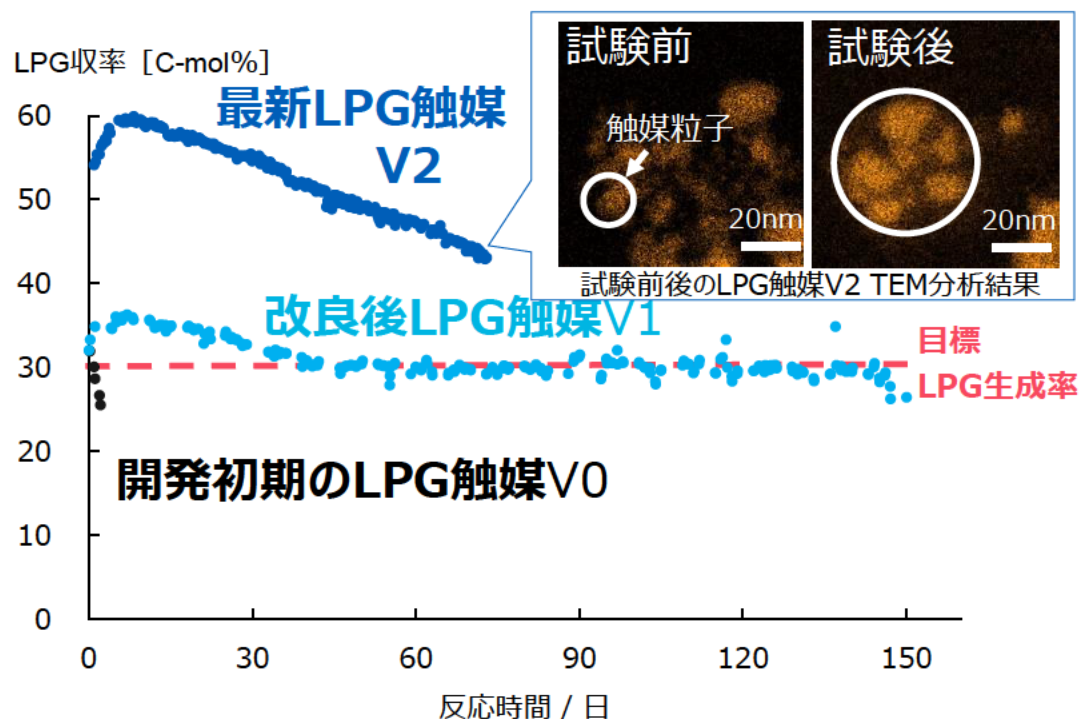
図1 LPG触媒の長期試験結果
