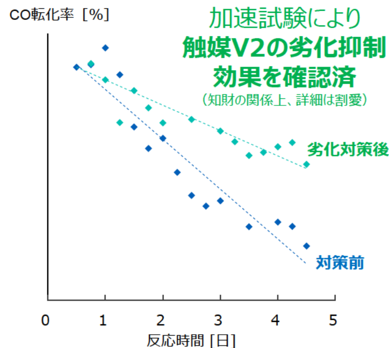
図2 LPG触媒V2の加速試験結果
