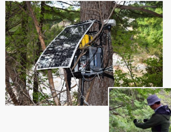
火山ガス
