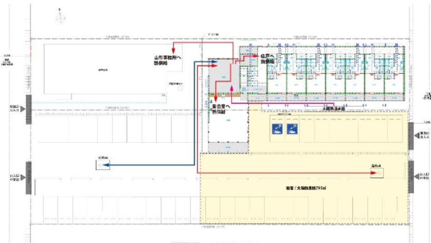
配置図 2025/11/06
