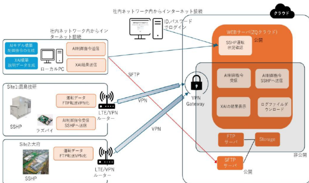
再エネ熱利用ヒートポンプ（SSHP）の遠隔計測用クラウド
