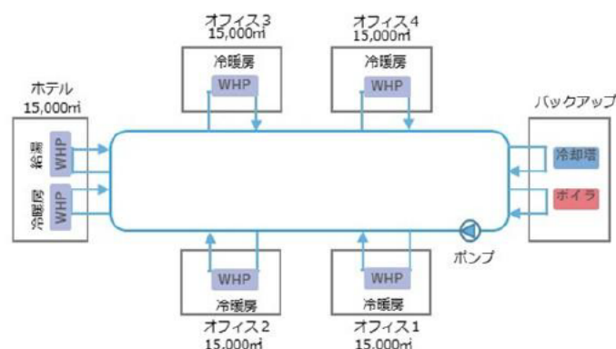
面的熱利用モデル
