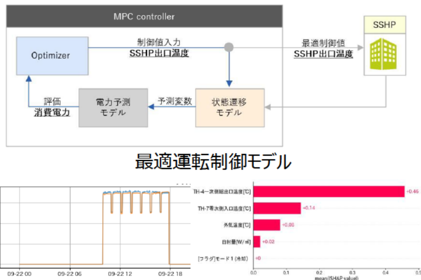
SSHP消費電力予測結果
