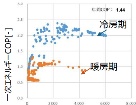
負荷と一次エネルギーCOPの関係(ダブルフープ)
