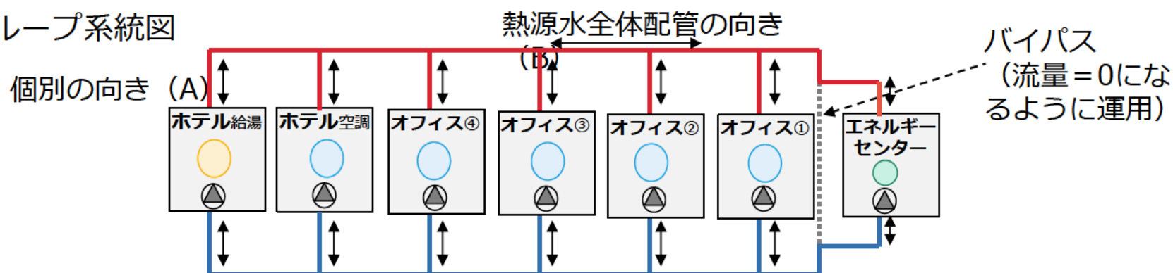
LCЕМ計算モジュール（夏期代表日）
