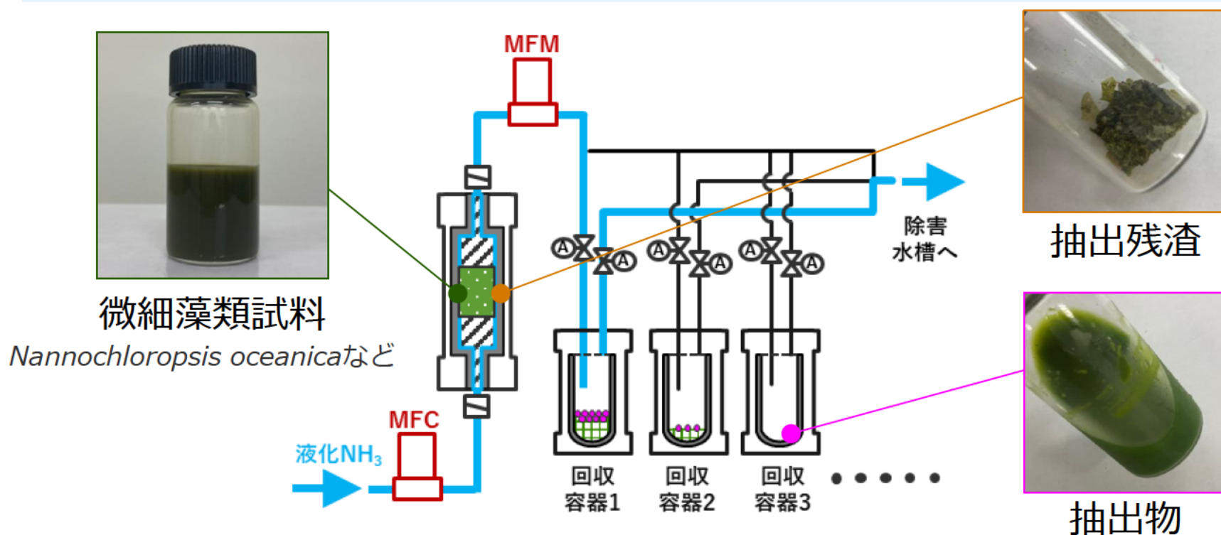
図 液化アンモニアによる抽出試験装置の概略系統
