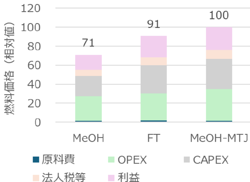
ベースケース (LHV基準*1)
