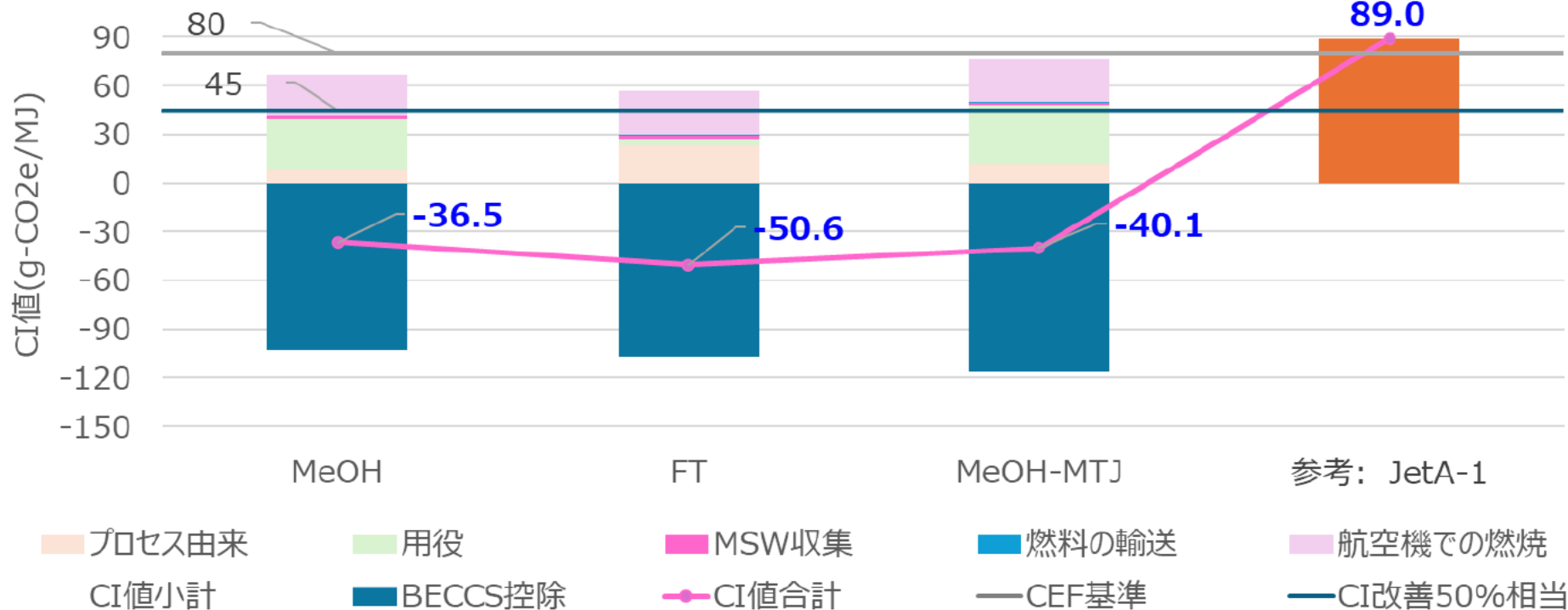
合成燃料 各製造ルートCI値比較
