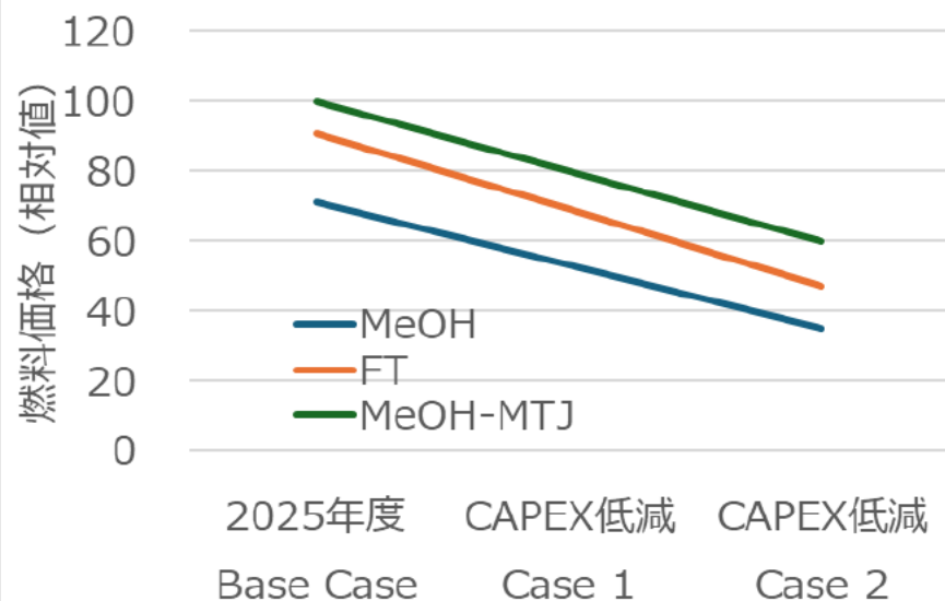
ガス化炉CAPEXの影響(LHV基準*1)
