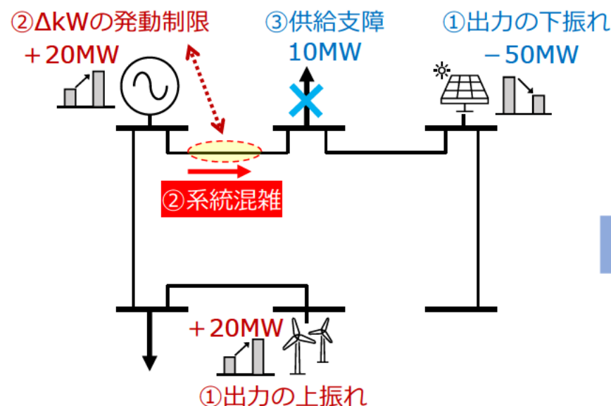
(a) ΔkWの発動制限による 供給支障の発生
