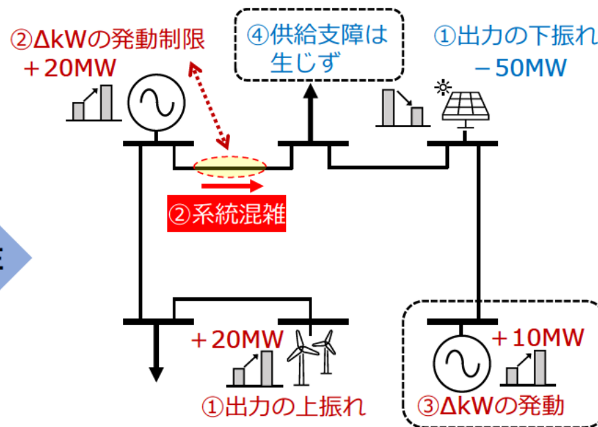
(b) ΔkWの追加調達による 供給支障の回避
