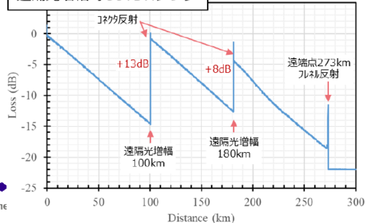
遠隔光増幅時COTDRグラフ
