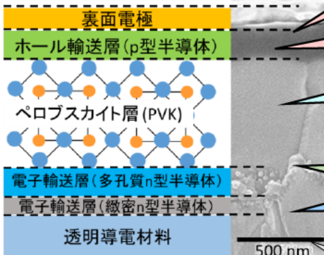
ペロブスカイト単接合太陽電池
