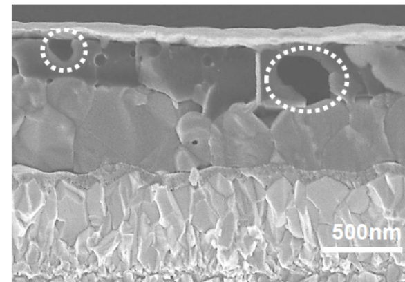
85°C試験、400時間後
