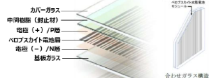
合わせガラス構造
