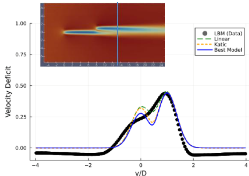
Trial Cのスタガード位置（2基めの風車は8D後方、 Y方向に0.5Dずれ）の後流プロファイル比較
