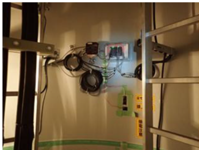
タワー部のひずみゲージ貼付状況
