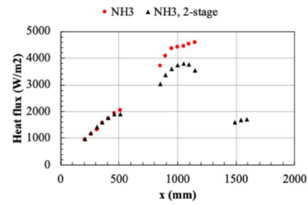
熱流束分布
