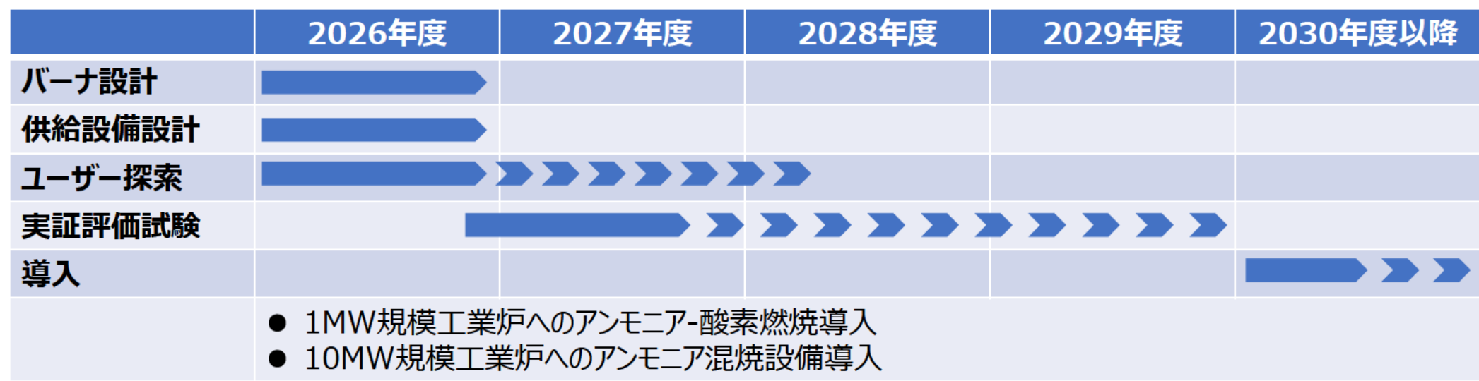
工業炉における燃料アンモニア燃焼技術の導入イメージ
