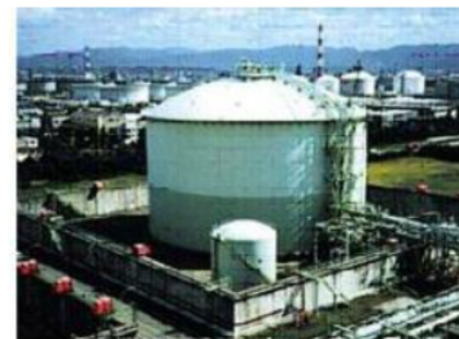
防液堤と大型平底円筒形 貯槽の例（LNG貯槽）
