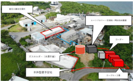
副生水素出荷設備整備イメージ
